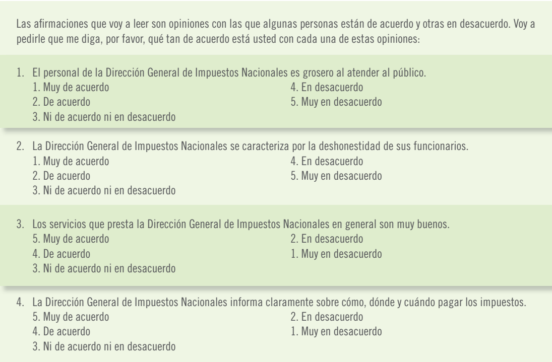
Figura 9.12 Muestra de una escala Likert.
