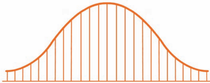
Figura 10.14 Distribución muestral de medias.
