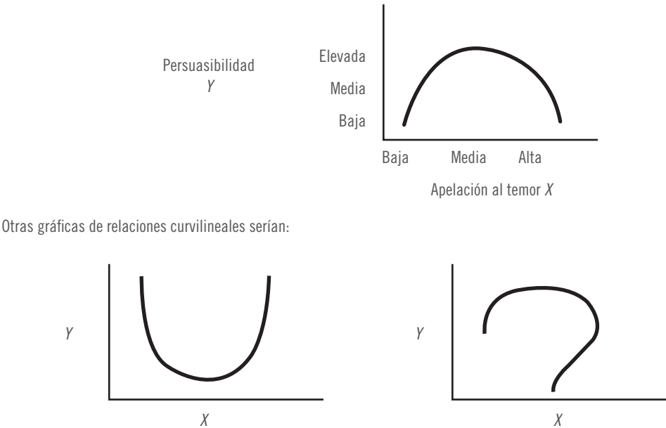
Figura 10.19 Ejemplos de relaciones curvilineales.
